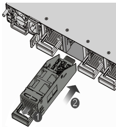
Figure 4: Installing a Fan Module
