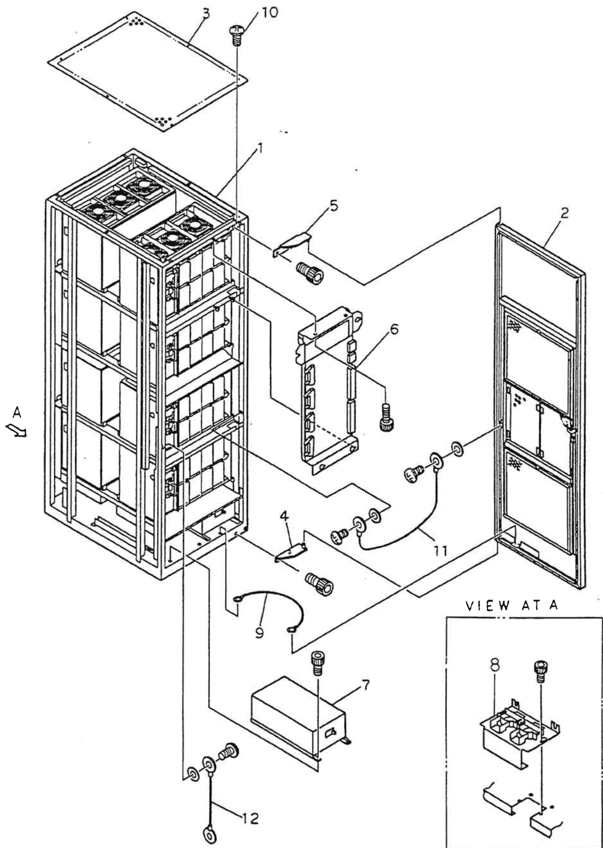
Fig. 1-2 DKU205 FINAL ASSY
