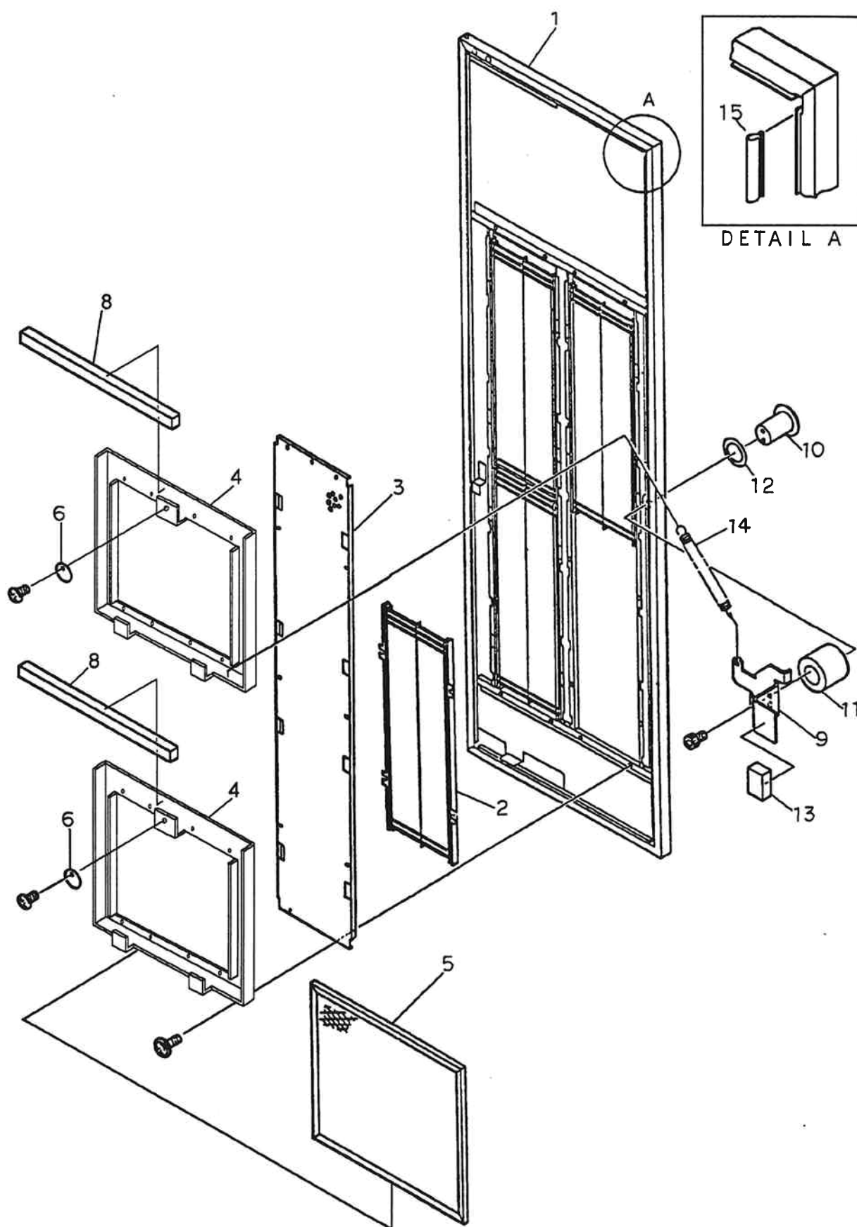
Fig. 1-4A DKU DOOR ASSY
