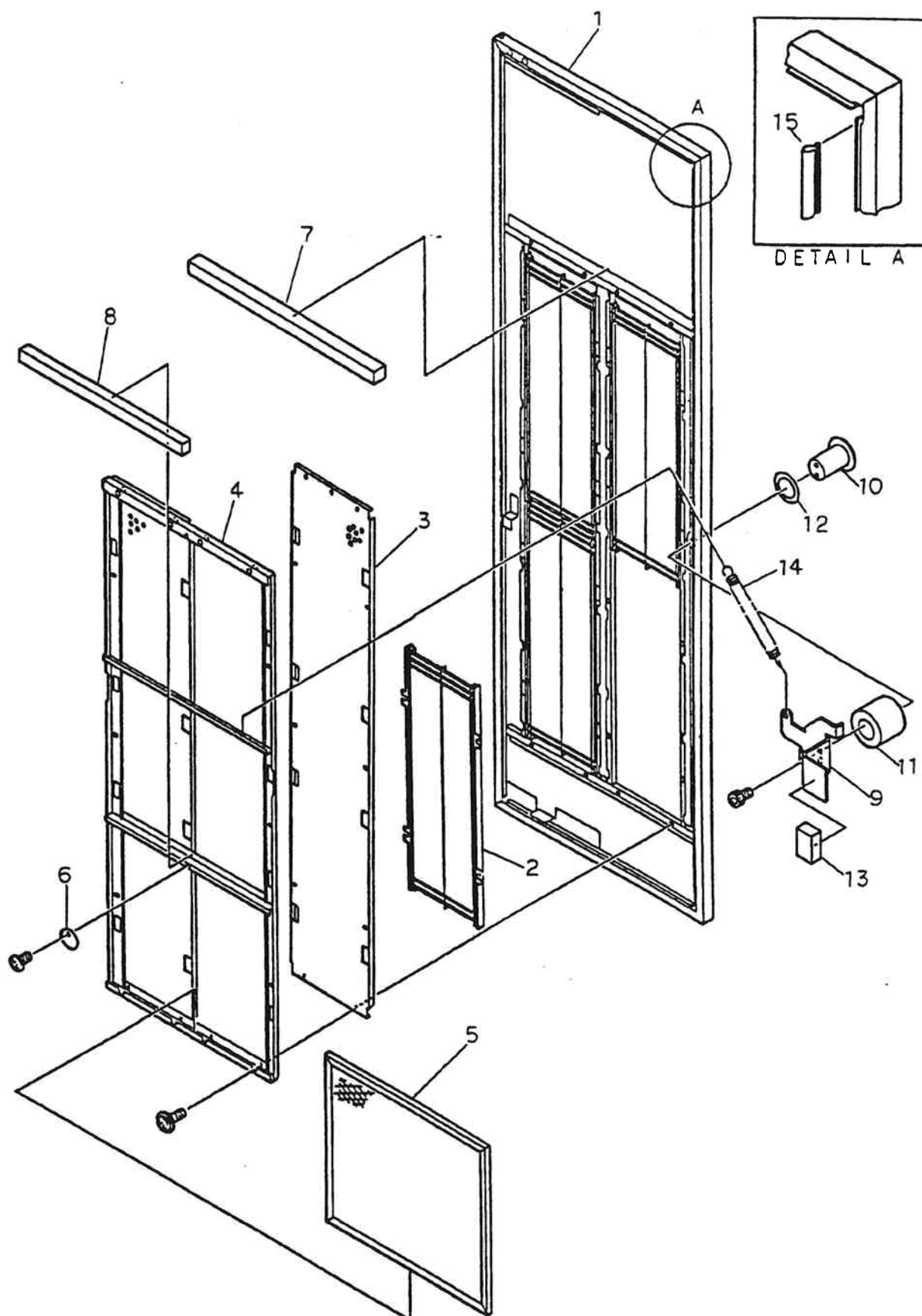
Fig. 1-4 DKU DOOR ASSY
