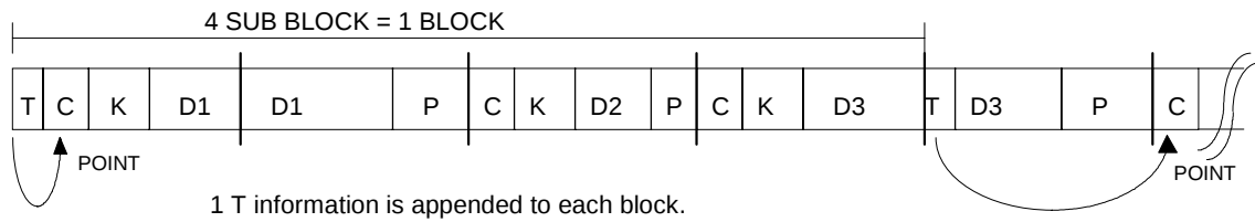
Fig. 3.3.2 Block Format
