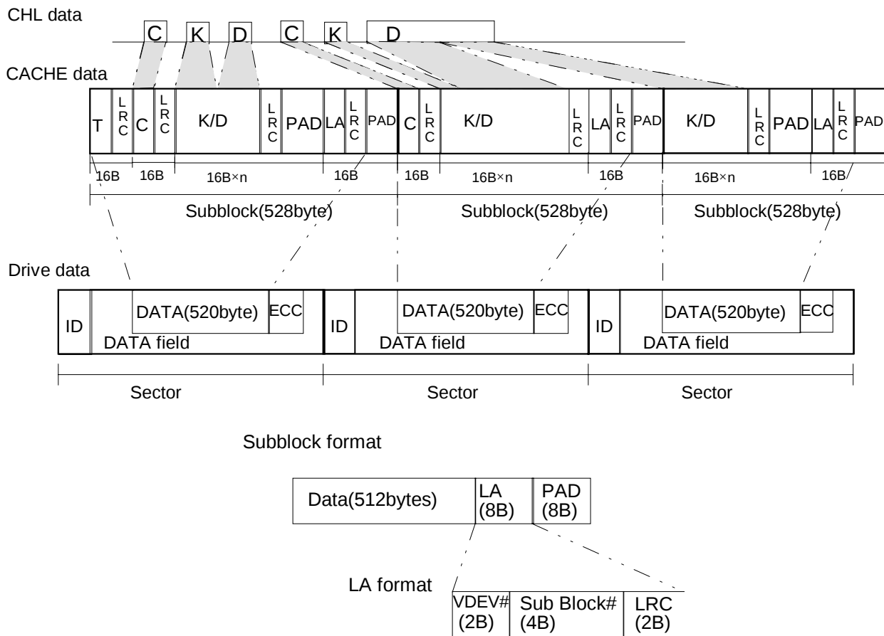
Fig. 3.3.1 Data Format
