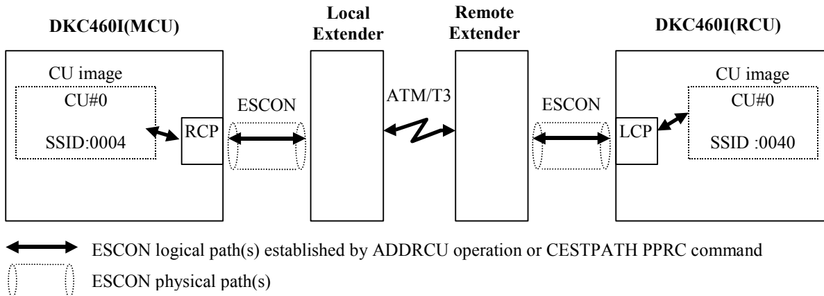
Fig 3.11.3-3 MCU:CU#0 &lt;--&gt; RCU:CU#0 (valid configuration)
