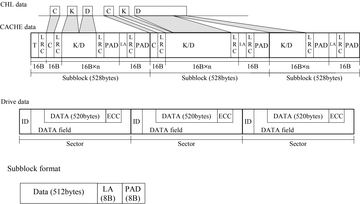
Fig. 3.3-1 Data Format
