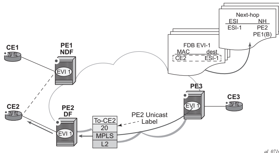
Figure 168 Backup PE
