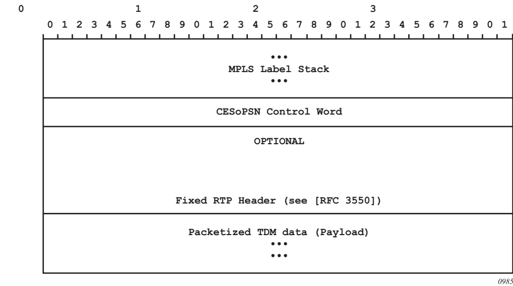
Figure 4 CESoPSN MPLS Payload Format
