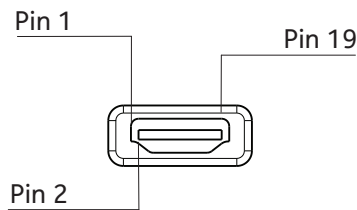
View A-A
