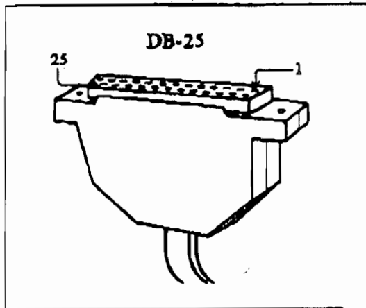
DB-25 PIN
