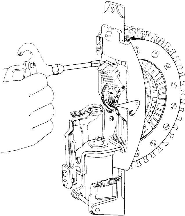
Fig. 9—206-, 209-, and Similar-Type Selectors
