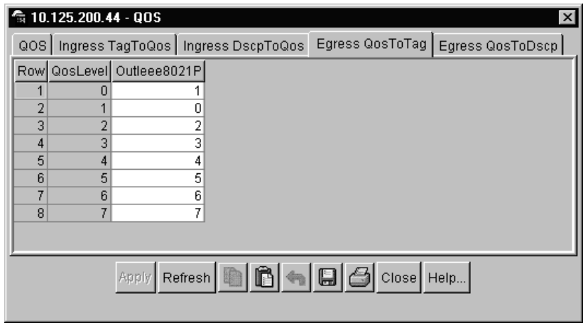
Figure 14 QOS dialog box—Egress QosToTag tab
