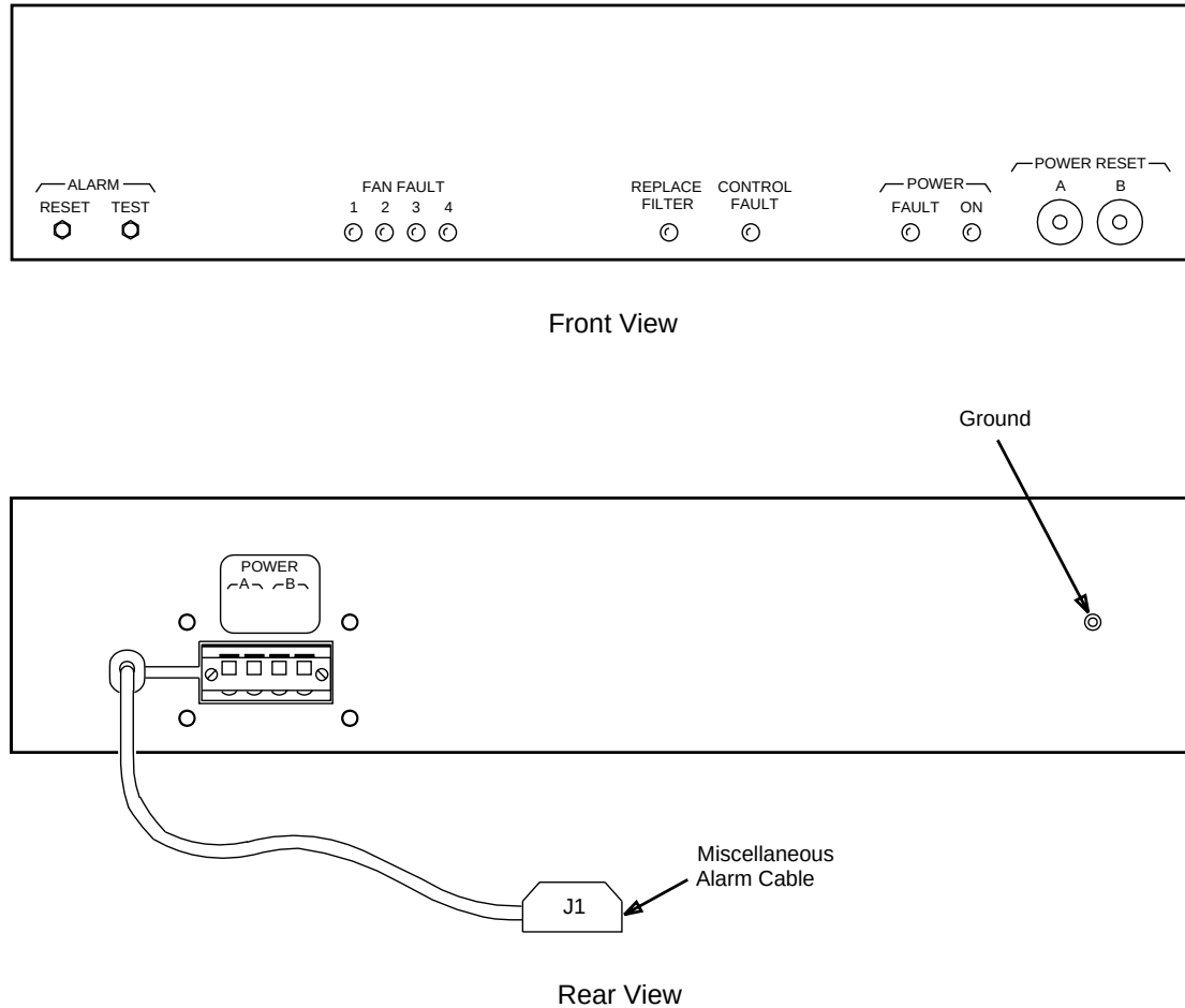
Figure 4-8. DDM-2000 Fan Shelf
