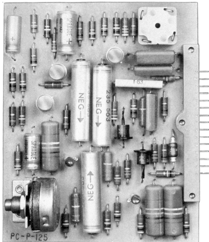
Fig. 4 — KS-16765, List 6 Amplifier
