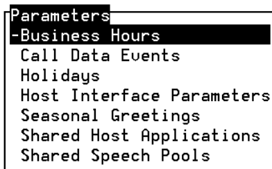
Figure 48. Parameters Menu
