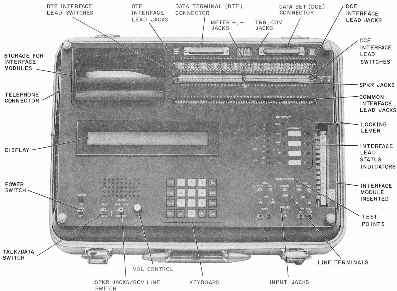
Fig. 1—921A Data Test Set—Front Panel
