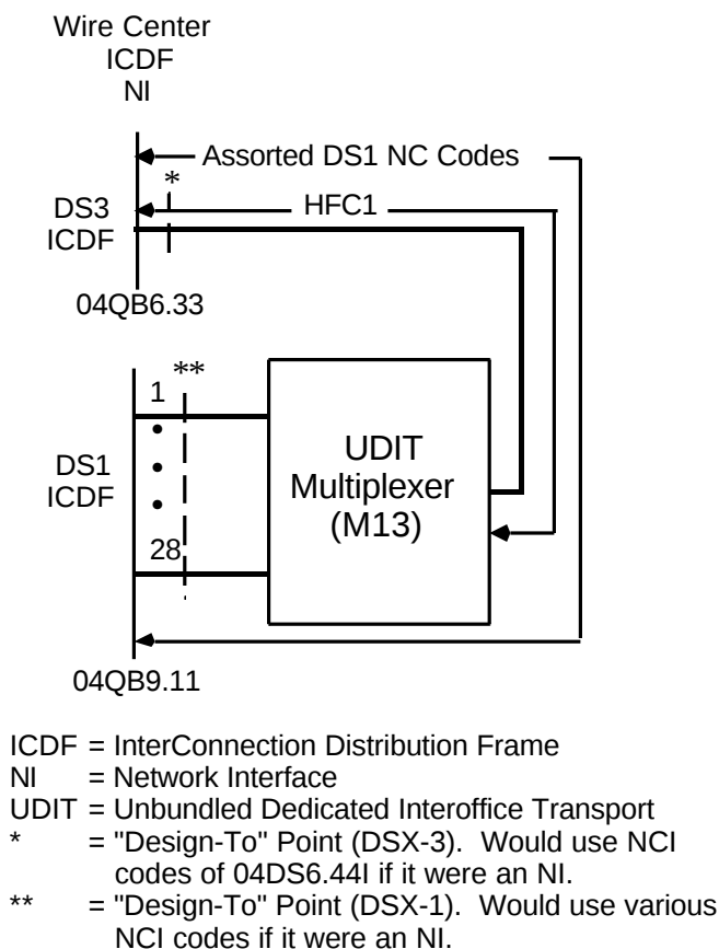
Figure B-3: Typical DS3 UDIT Multiplexer UNE
