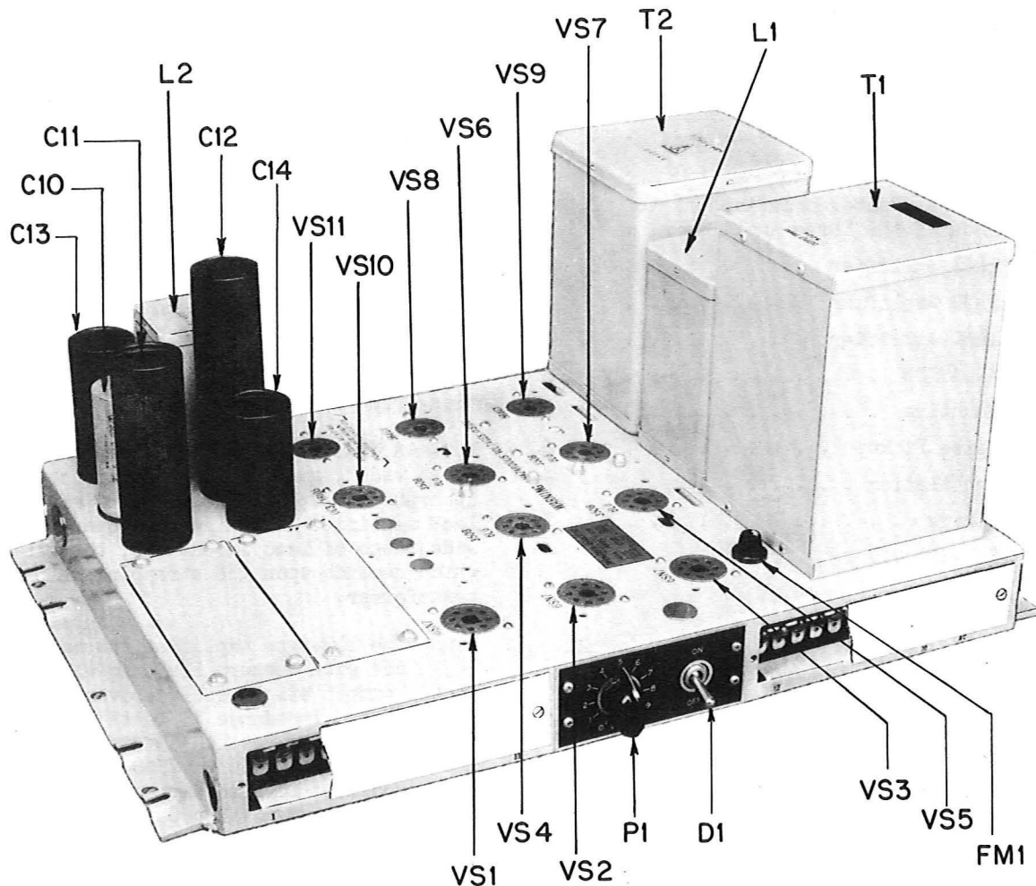
Fig. 1 - 143A Amplifier
