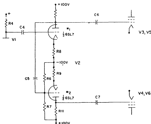
Fig. 3—Phase Inverter Schematic
