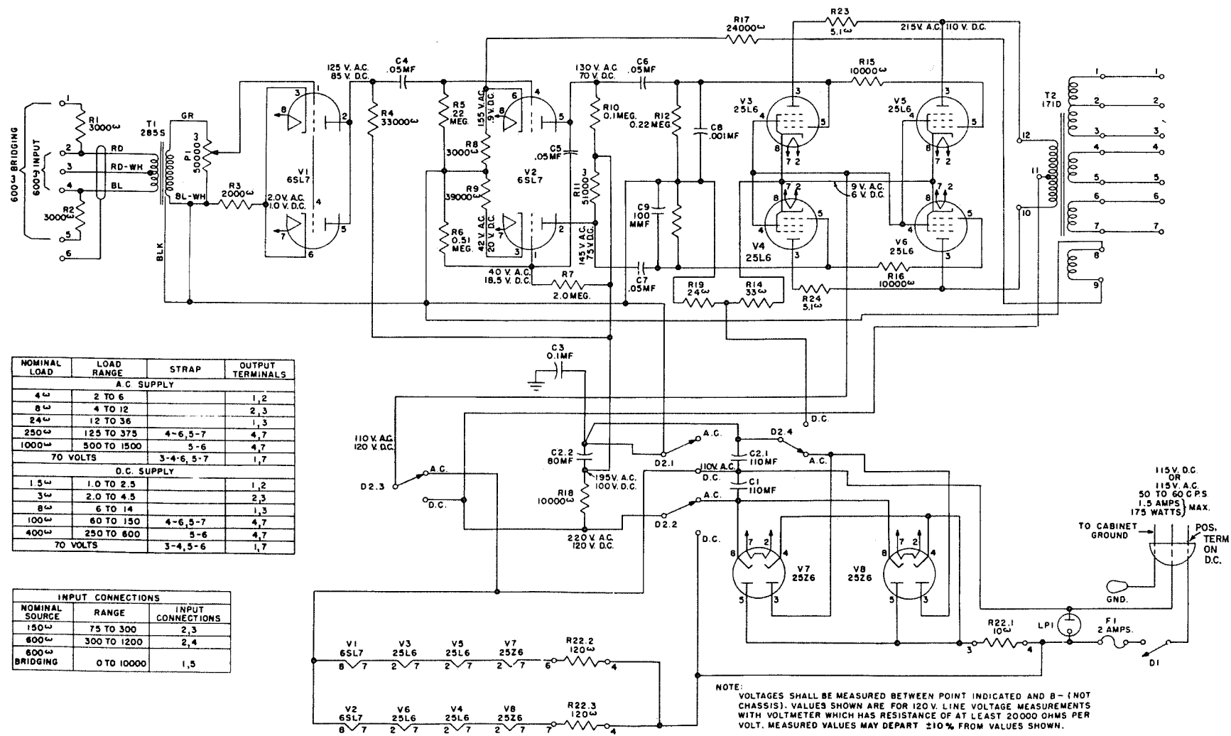
Fig. 2—140A Amplifier Schematic
