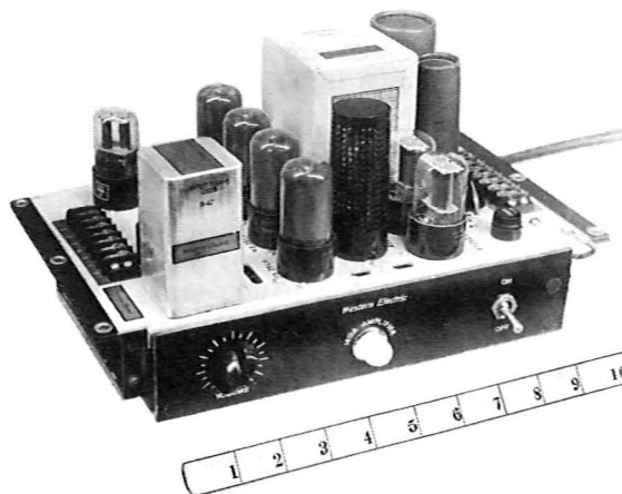
Fig. 1—140 Amplifier
