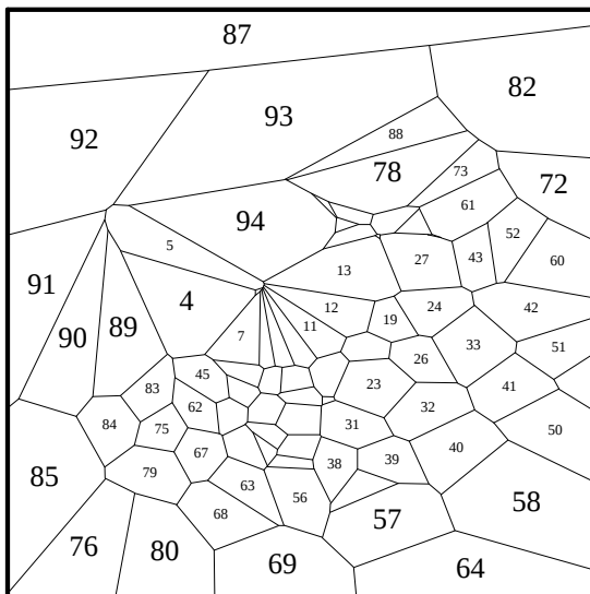
Fig. 70: dual proj. it. 13, v = \text{center}
