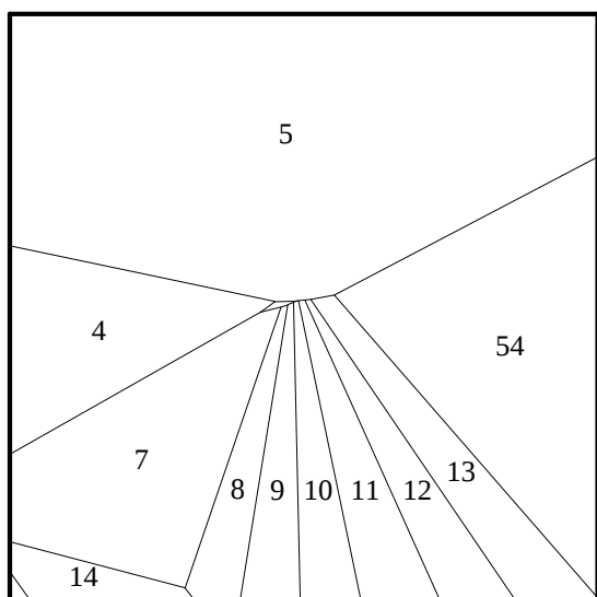
Fig. 110: pr. proj. it. 10, v = \text{center}
