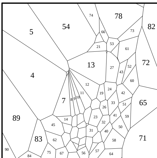
Fig. 122: pr. proj. it. 16, v = \text{center}
