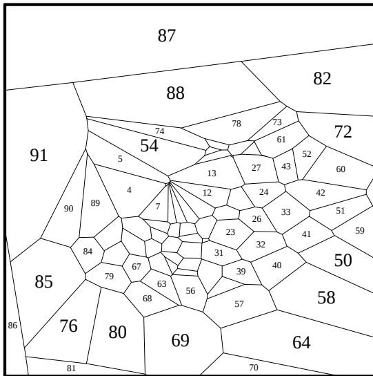
Fig. 130: pr. proj. it. 20, v = \text{center}
