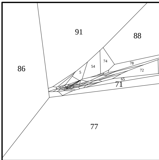
Fig. 132: pr. proj. it. 21, v = \text{center}
