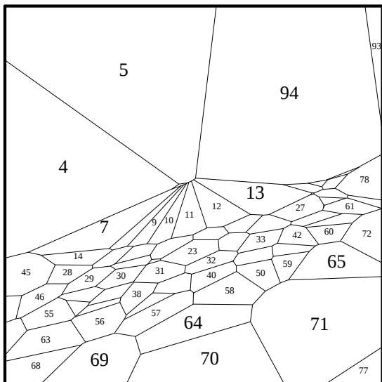
Fig. 54: dual proj. it. 5, v = \text{center}
