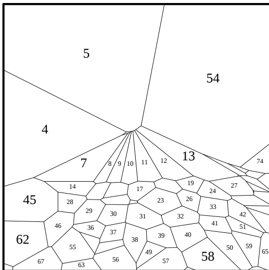
Fig. 114: pr. proj. it. 12, v = \text{center}
