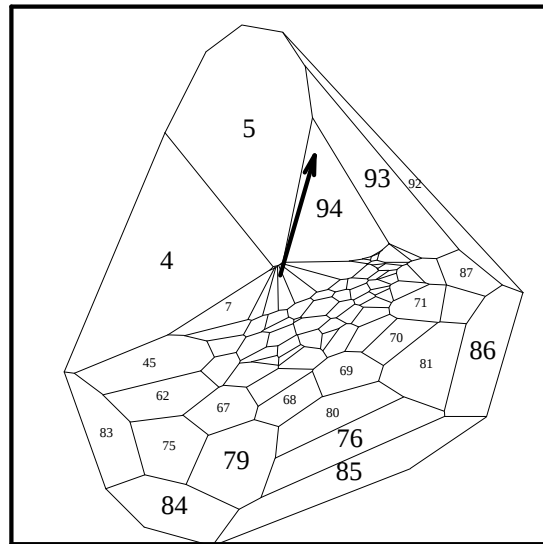
Fig. 49: dual proj. it. 2, v = \text{center} + (.2, 0, 0)
