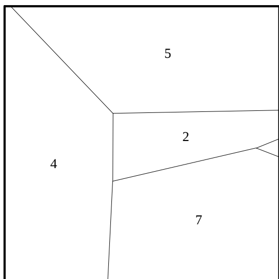
Fig. 102: pr. proj. it. 6, v = \text{center}
