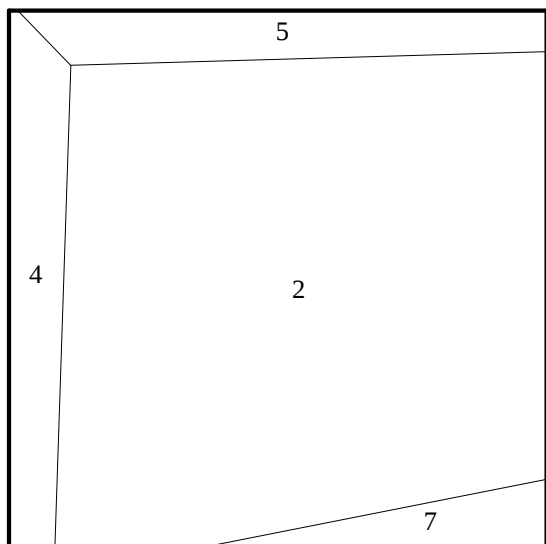
Fig. 100: pr. proj. it. 5, v = \text{center}
