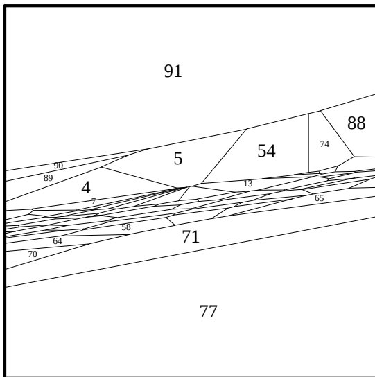
Fig. 126: pr. proj. it. 18, v = \text{center}
