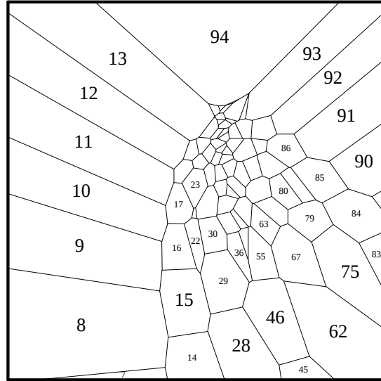
Fig. 137: pr.p.it. 2, d = \text{behind} , nat. vars.
