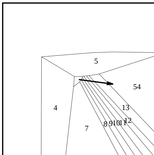
Fig. 107: pr. proj. it. 8, v = \text{center} + (.1, 0, 0)
