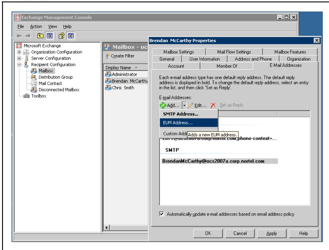
Figure 123 UM Address
