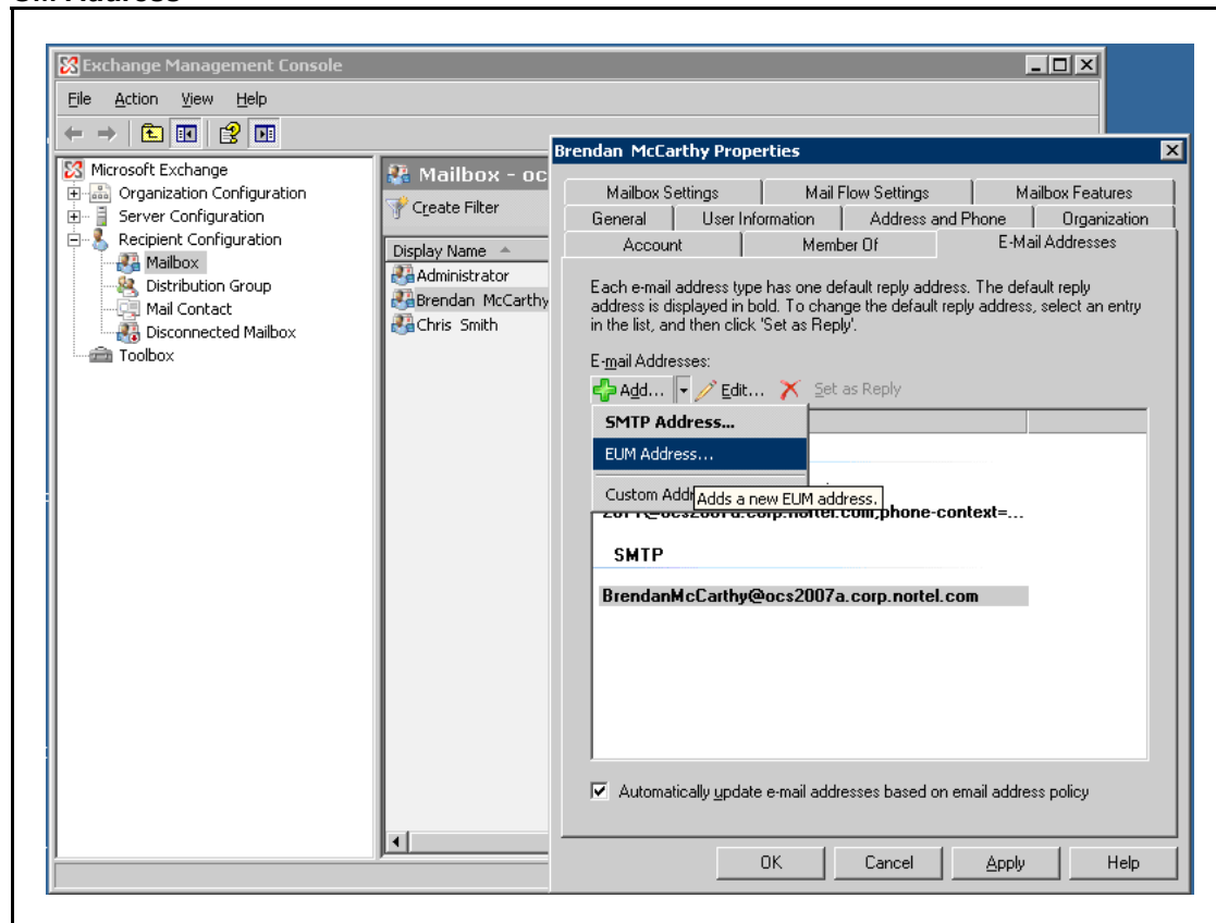
Figure 128 UM Address
