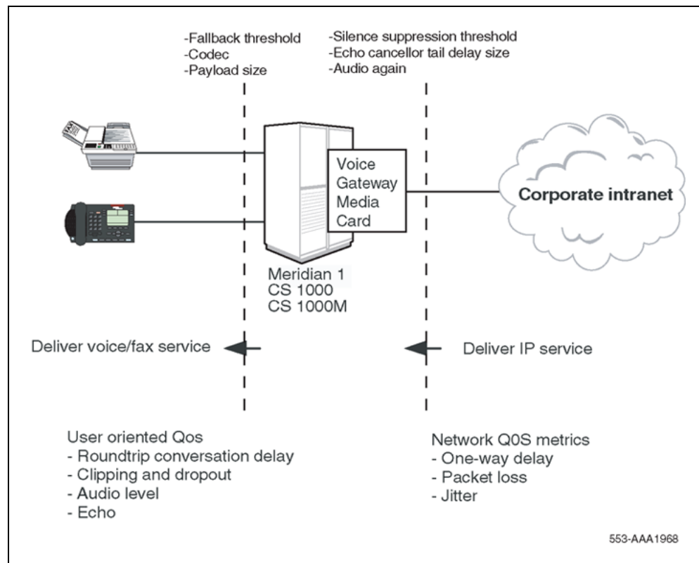
Figure 19 QoS parameters
