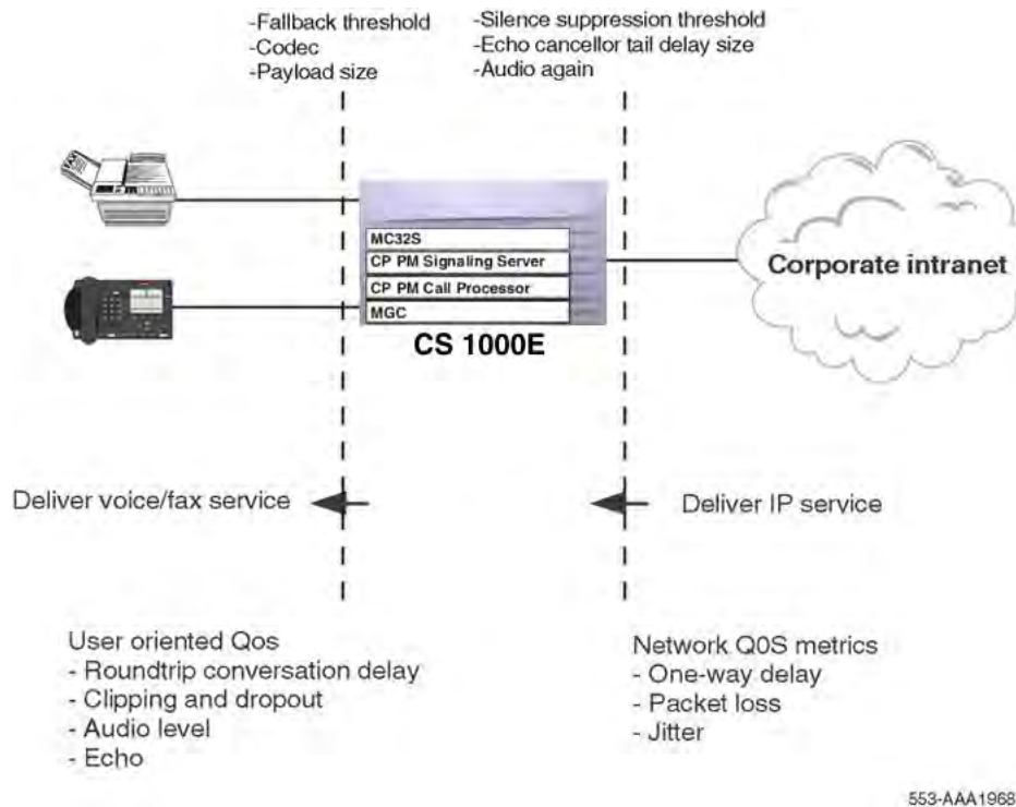
Figure 28: QoS parameters
